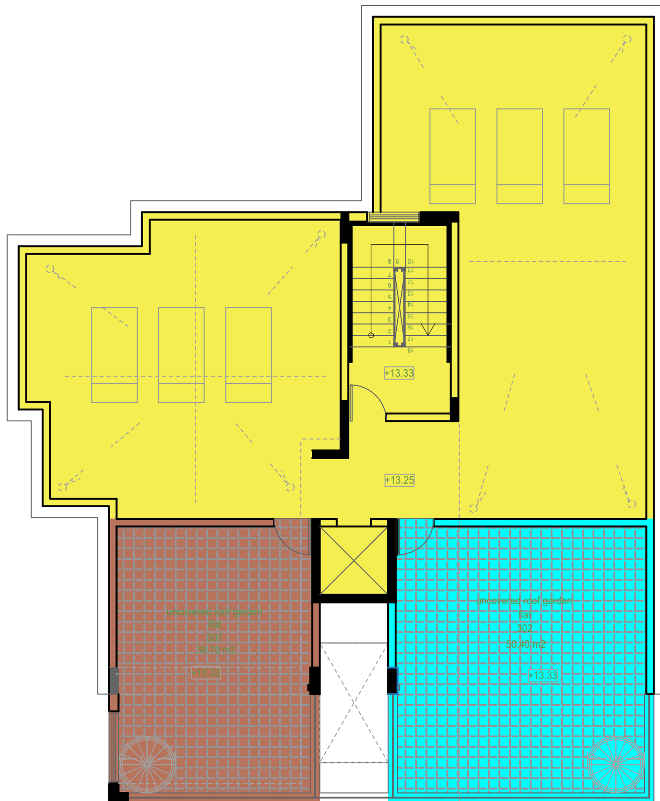
ΚΑΤΟΨΗ ΟΡΟΦΗΣ
